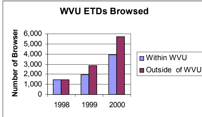
Figure 5 ETD Browsers
